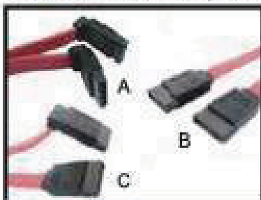
A: E284008292 SATA CABLE 90/90 B: E284008170 SATA CABLE 180/180 C: E284008293 SATA CABLE 90/180
