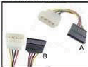
A: NA100-008-006 POWER CABLE FOR SERIAL ATA HDD B: SF217-008-305 0.3M SERIAL ATA/150 CABLE 180-180, L=0.3M
