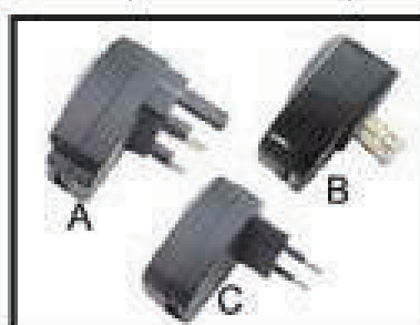
A,B,C USB AC POWER ADAPTOR (CHARGER) INPUT : 90-240 VAC OUTPUT : 5.2V,500MA COLOR : BLACK - WHIT - PINK SAFETY : PSE/UL/CE
