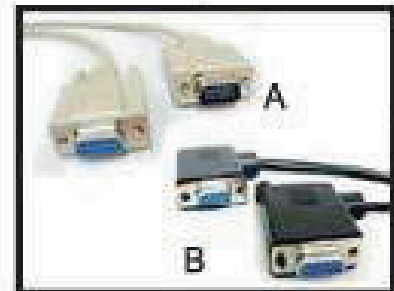
A: Q217-021-077_2M DB9M TO DB9F 38P*9C+DW+AL OD:5.0 B: Q153-021-078 DB9F/DB9F (R/A) CABLE, L=2.44 MM
