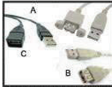
A: Q153-025-161 USB AM/AF (WNU) CABLE B: Q150-025-019 2M USB AM/BF CABLE C: S284-025-248 USB 2.0 AM/AF CABLE COLOR: BEIGE/BLACK/GRY
