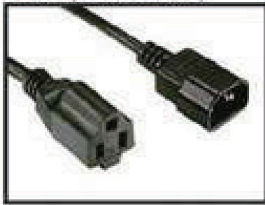
Item No. : E012018443_1.8M SJT 16/3 SJT 14/3,L=1.8M (UL & C-UL APPROVAL)
